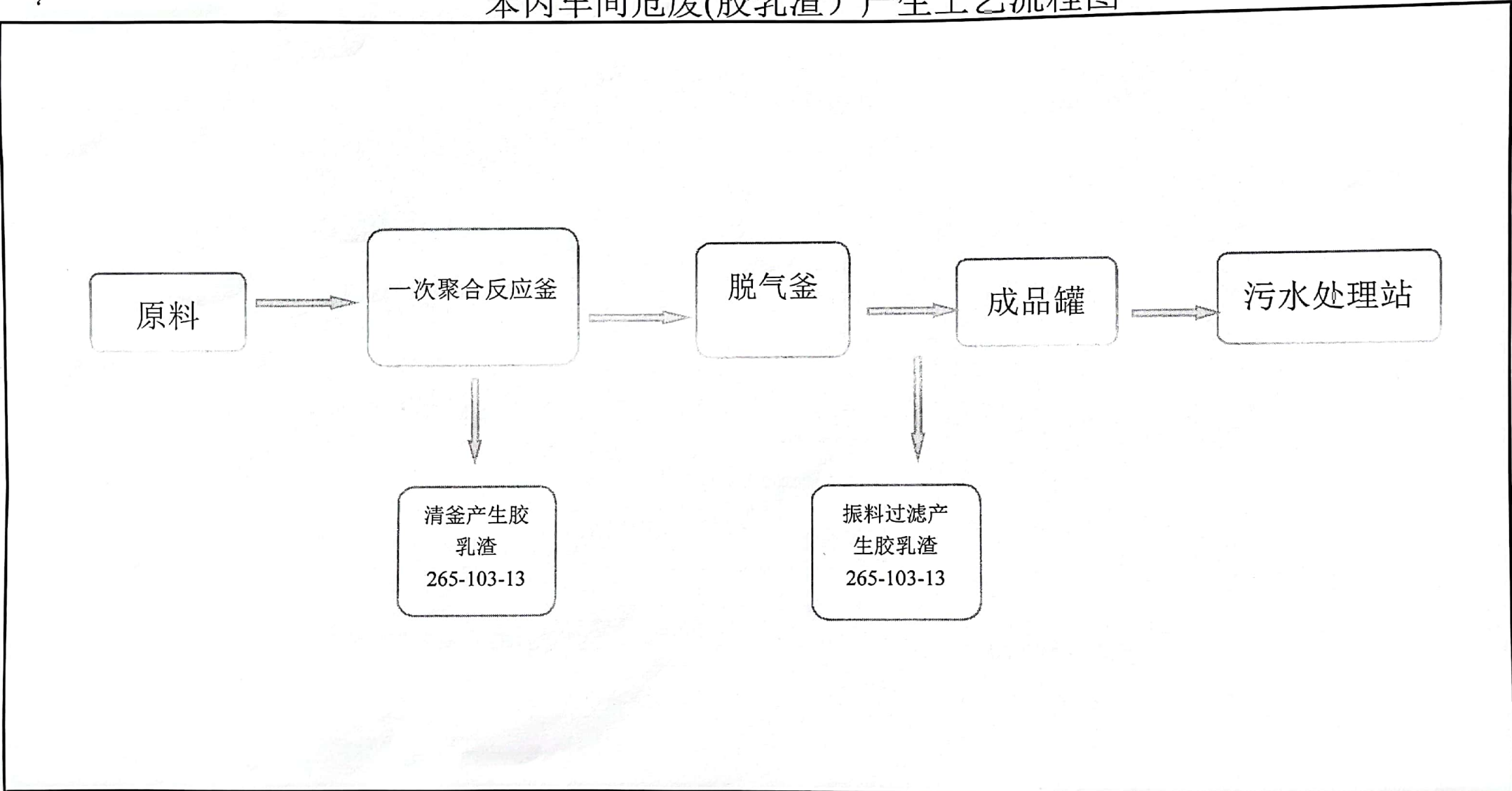
苯丙车间危废(胶乳渣)产生工艺流程图
